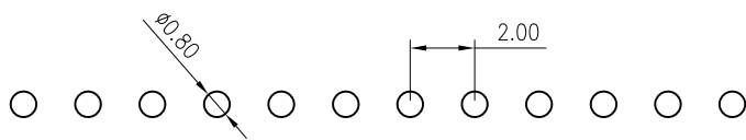
P.C.B LAYOUT
