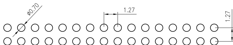
P.C.B LAYOUT
