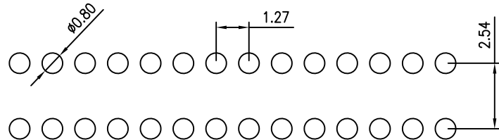
P.C.B LAYOUT
