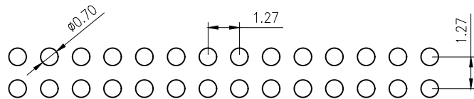
P.C.B LAYOUT
