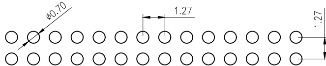
P.C.B LAYOUT
