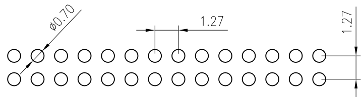
P.C.B LAYOUT
