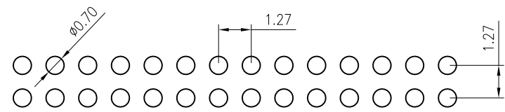
P.C.B LAYOUT
